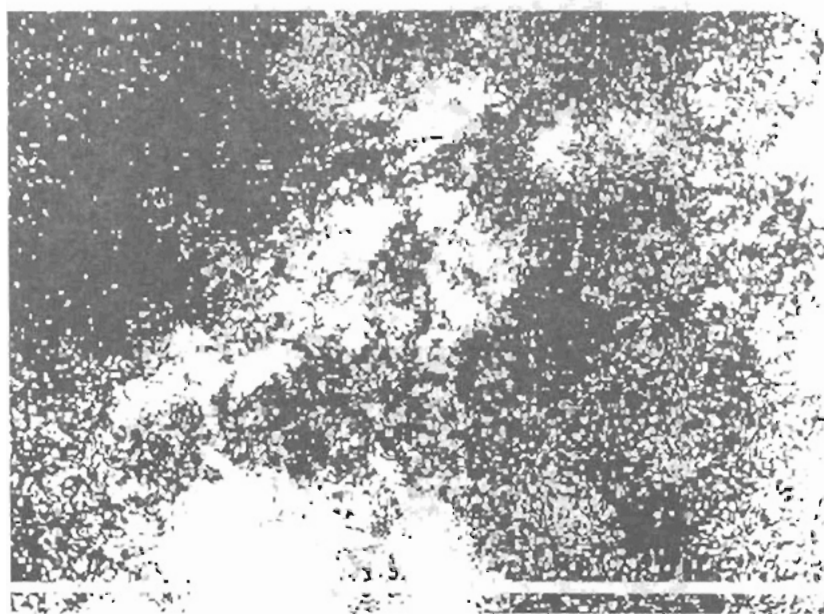
Hình 43: Tinh Vân một phần dải Ngân Hà
