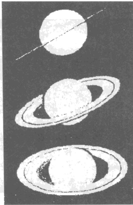
Hình 53: Sao Thổ (Saturn) và vành đai của nó (Nhìn theo các góc độ khác nhau)
