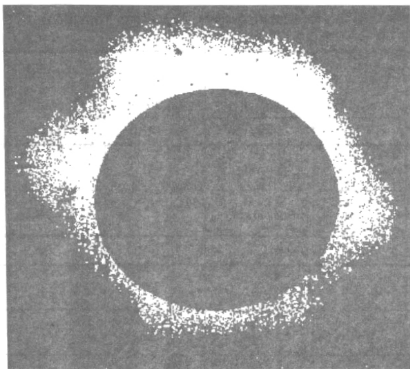
Hình 47: Nhật thực và vòng Nhật quang
