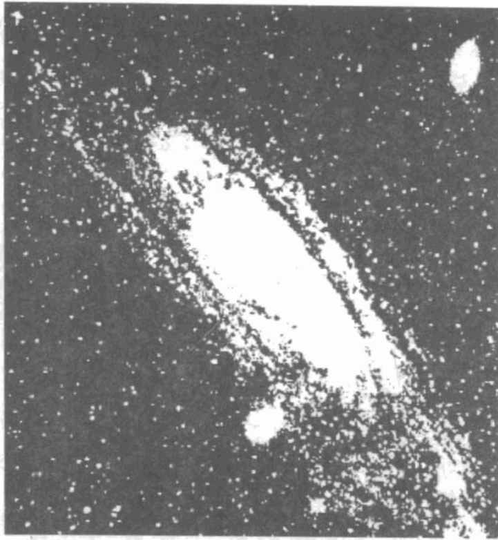
Hình 44: Tinh vân thiên hà Andromede
