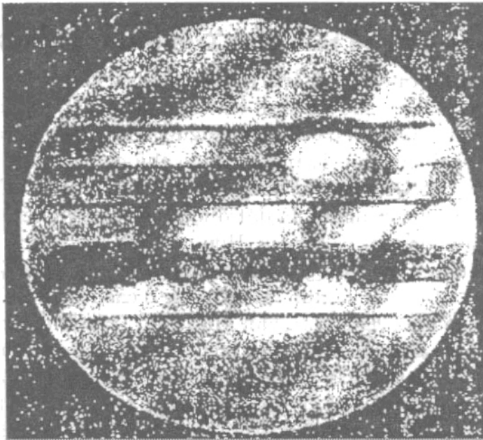
Hình 52: Sao Mộc (Jupiter)
