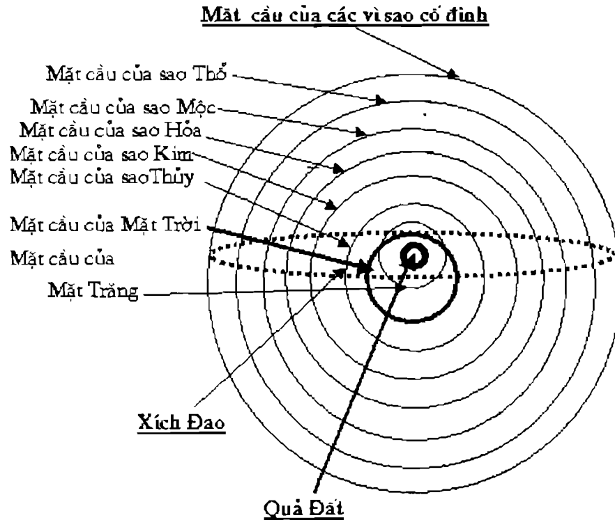
Hình 58: Mô Hình Vũ Trụ “Địa tâm” cổ đại (Ph. Tây) (của Ptolémée)
