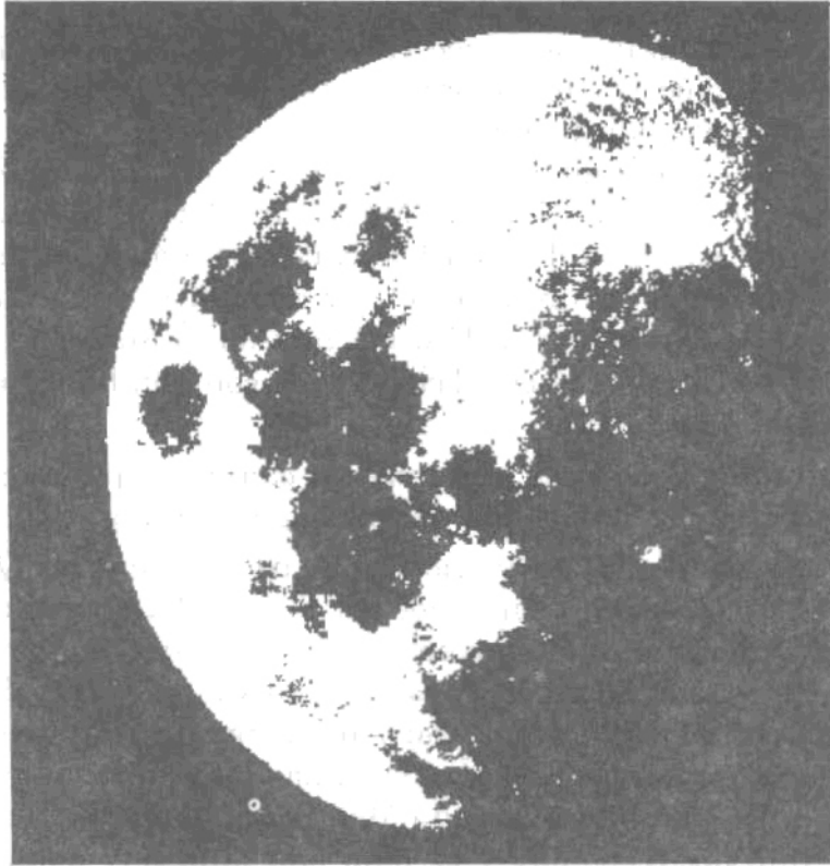
Hình 54 : Mặt Trăng. (Ngày thứ 11 sau tuần Trăng tròn)
