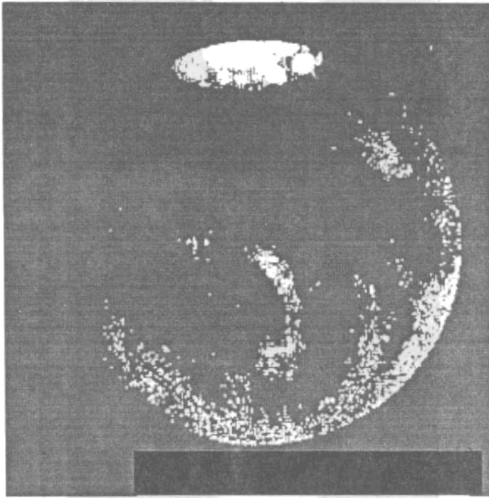
Hình 51: Sao Hỏa (Mars)
