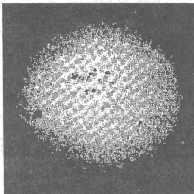
Hình 46: Các vết đen trên Mặt Trời
