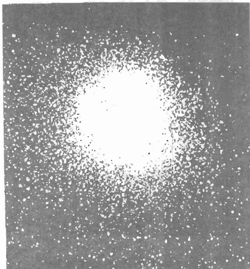
Hình 42: Tinh vân M13 (trong chòm Hercules)
