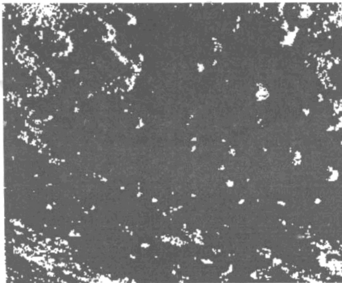
Hình 50: Bề mặt Sao Thủy (Mercure)
