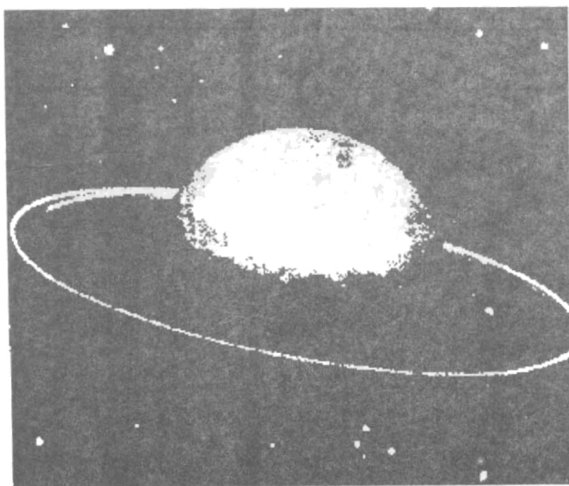
Hình 48: Sao Thiên Vương (Uranus)
