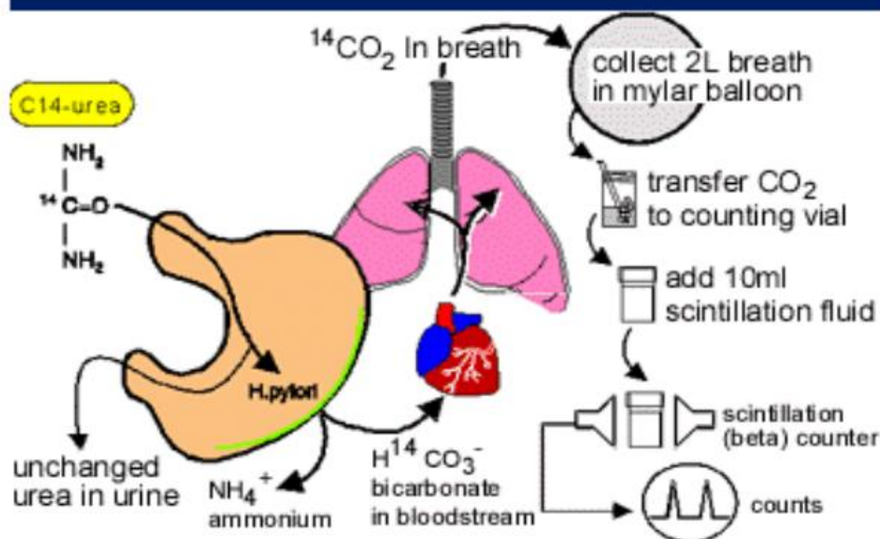
Hình 22. Tét thở urê mang đồng vị phóng xạ C 14
