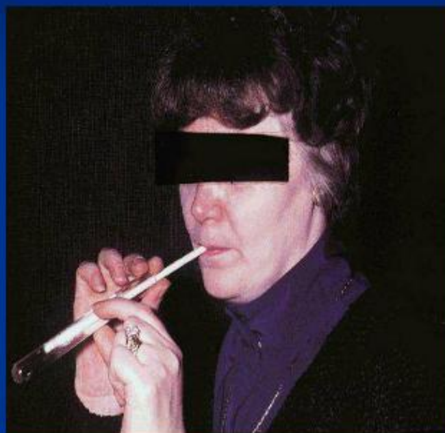
Hình 21. Test thở Urê C-13
