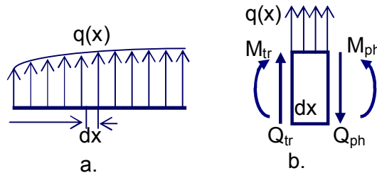
Hình 1.7. Phân tử của thanh chịu tải phân bố
