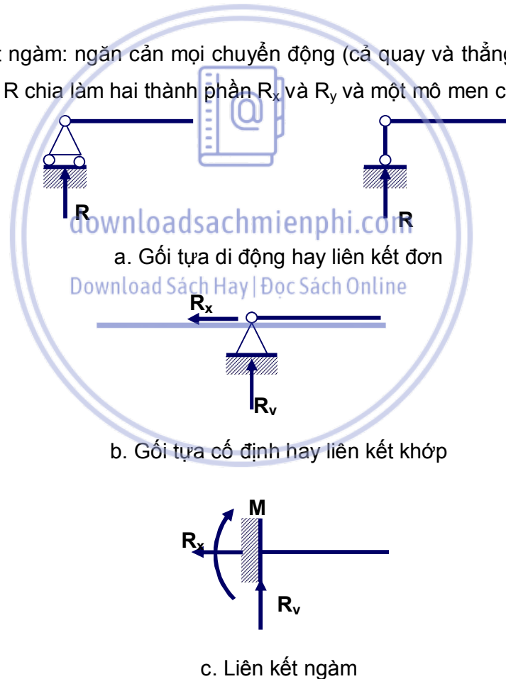
Hình 1.1. Biểu diễn các liên kết thường gặp trong trường hợp phẳng
