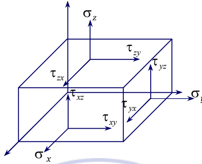
Hình 2.3. Thành phần ứng suất tại phân tố
