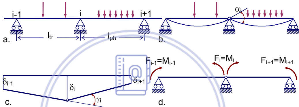
Hình 11.6. Thiết lập phương trình cho gối i
