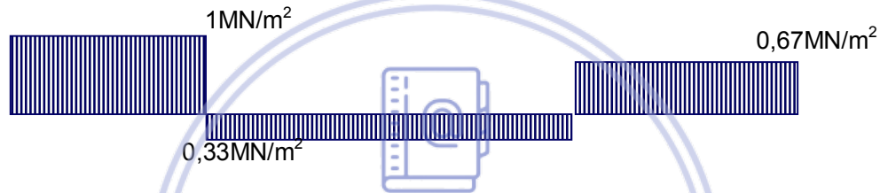
Hình 5.5. Biểu đồ ứng suất của thanh chịu lực dọc trục trên hình 5.2a
