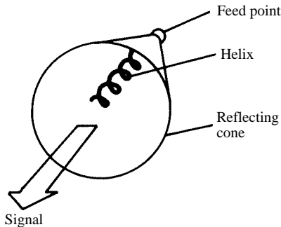
helicone
