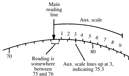
vernier, 1
