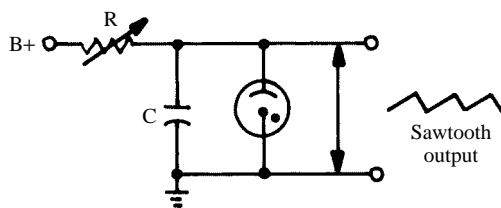
gas-tube oscillator
