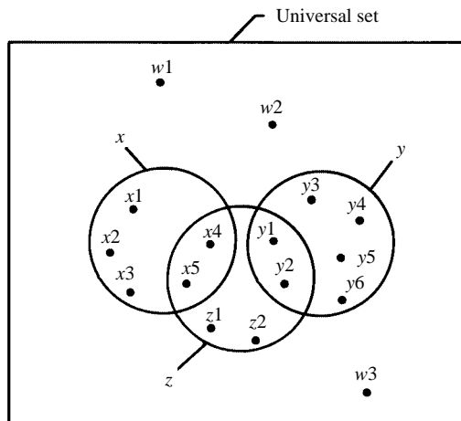
Venn diagram
