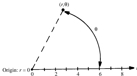
polar coordinates
